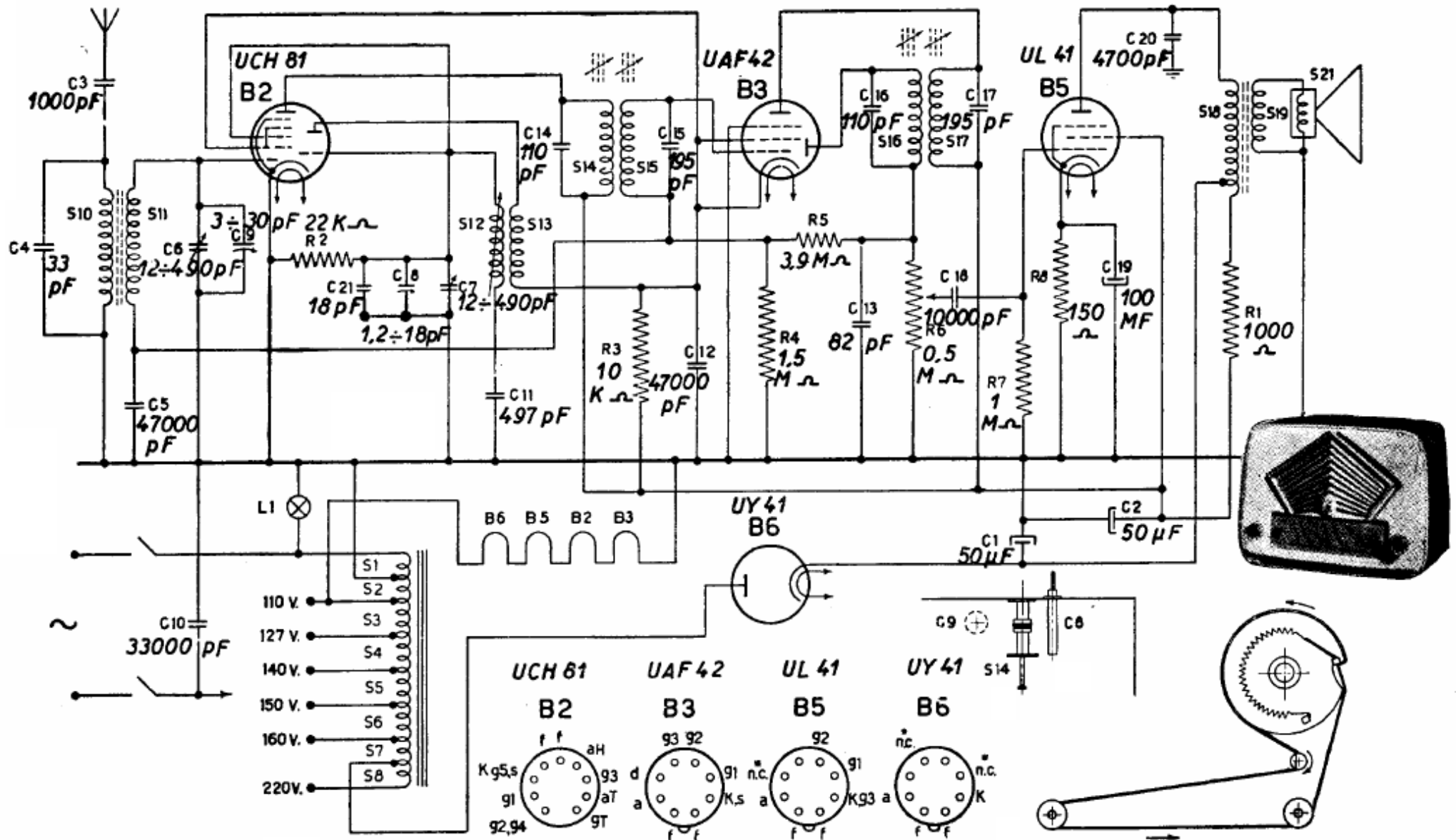
PHILIPS RADIO - Mod. BI. 140 A. Gamma onde medie. Media frequenza 468 kc/s. Tensione primo condensatore elettrolitico VC1 = 180 V, al secondo elettrolitico VC2 = 155 V. Corrente totale 72 mA. Consumo totale 30 watt. Tensione totale filamenti = 104 V.
